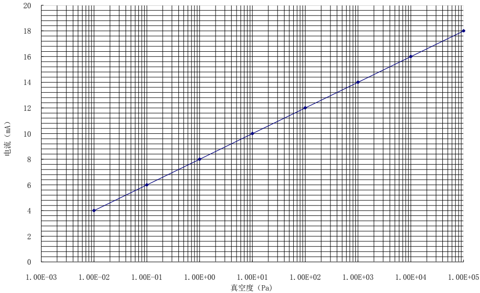
DZA1真空计真空度-电流输出曲线
