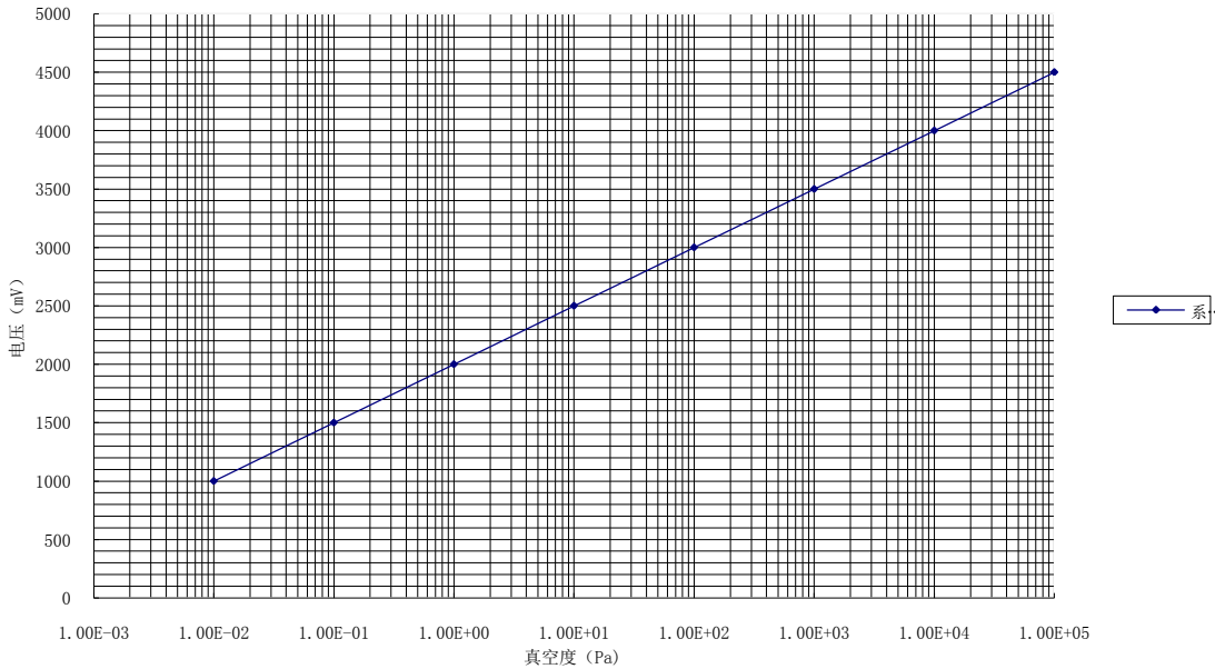
DZA1真空计真空度-电压输出曲线
